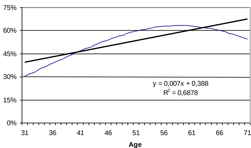
Fig. 12 : Mortalité des fumeurs par rapport à la population des fumeurs (hommes)
