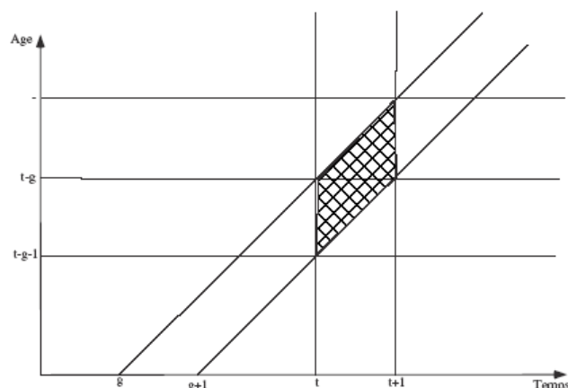
Fig. 7 : Identification des décès dans la génération g l'année t
