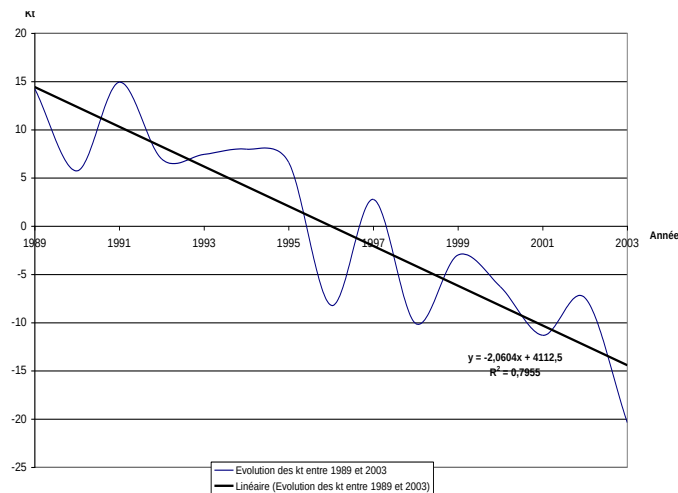
Fig. 17 : Évolution de la tendance temporelle
