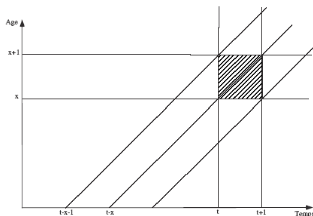
Fig. 4 : Identification des décès à l'âge x l'année t
