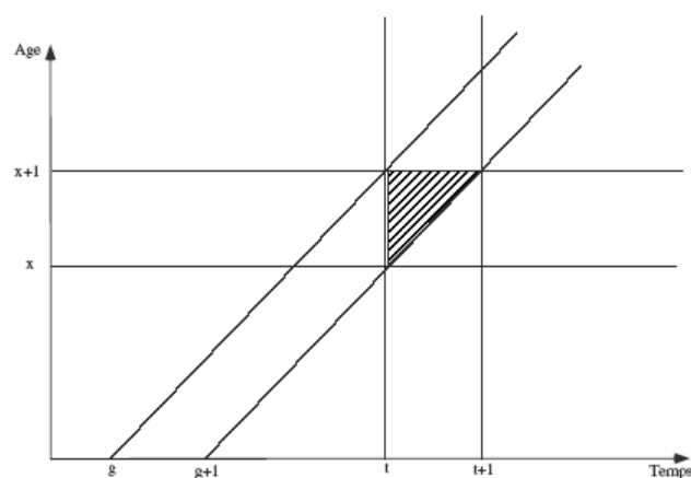
Fig. 6 : Identification des décès à l'âge x l'année t dans la génération g
