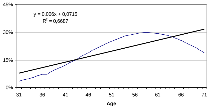
Fig. 13 : Mortalité des non-fumeurs par rapport à la population générale (hommes)
