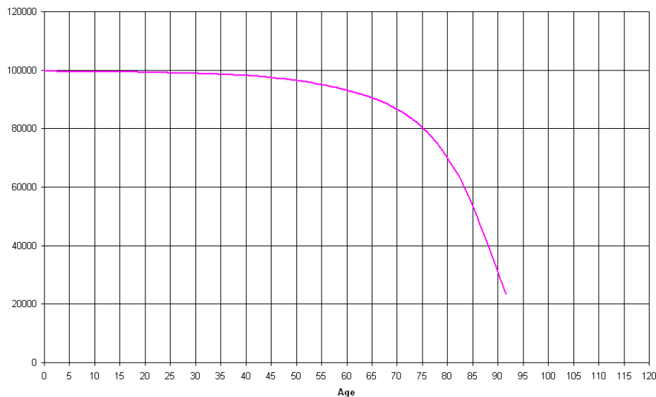
Fig. 2 : Représentation de la fonction de survie
