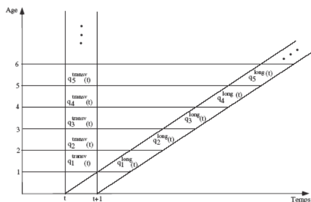
Fig. 8 : Mortalité longitudinale et mortalité transversale
